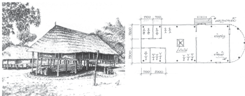
ภาพที่ 7 เรือนเผ่าตะไถ่ เมืองตะไถ่ แขวงสาละวัน
