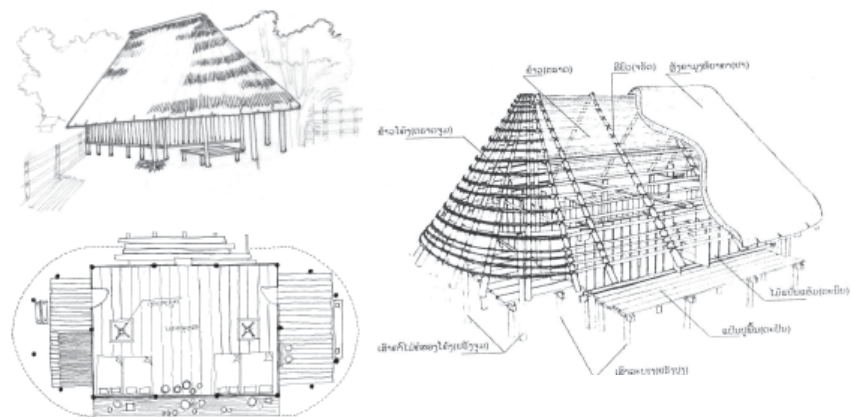
ภาพที่ 8 เรือนเผ่าเตี๋ยง เมืองดากัง แขวงเซกอง
