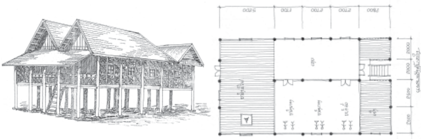
ภาพที่ 2 เรือนลาวลุ่ม เวียงจันทน์
