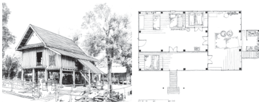
ภาพที่ 1 เรือนลาวลุ่ม หลวงพระบาง บ้านเมืองขาย เมืองหลวงพระบาง แขวงหลวงพระบาง
