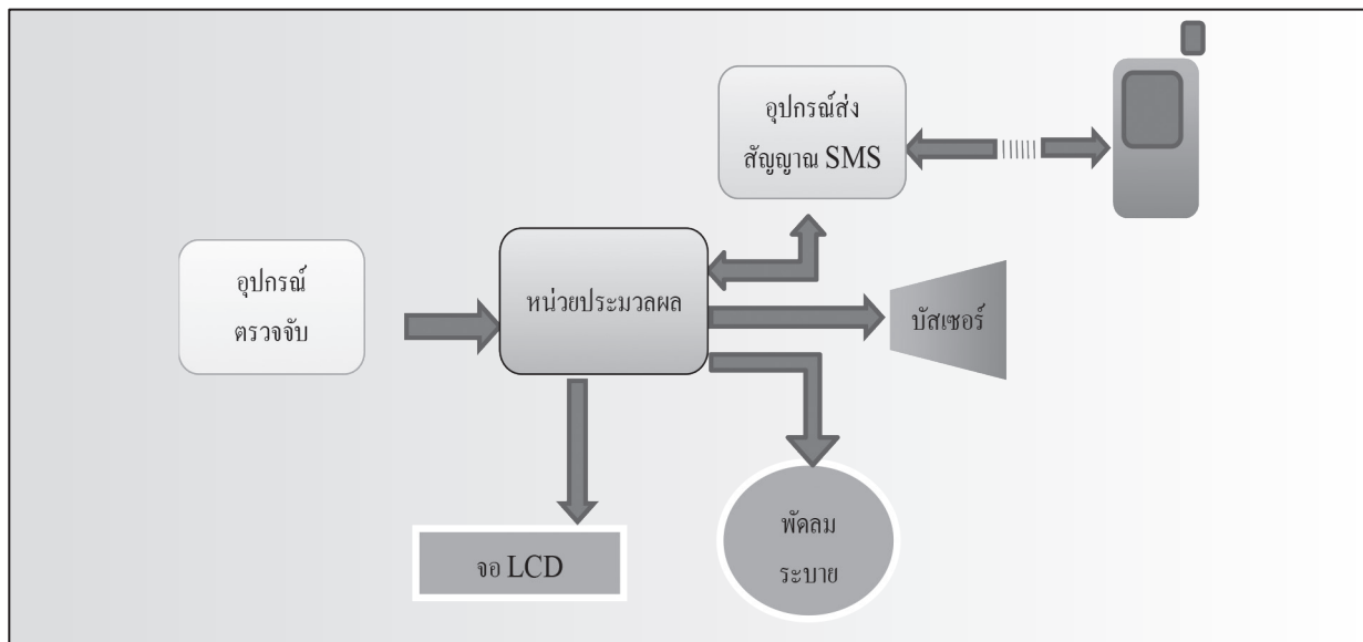
รูปที่ 2 บล็อกไดอะแกรมการทำงานของระบบการตรวจจับปริมาณก๊าซแอลพีจีในห้องครัวด้วยไมโครคอนโทรลเลอร์พร้อมระบบส่งสัญญาณเตือนภัยการออกแบบวงจรระบายอากาศ
