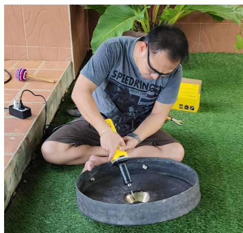
ภาพที่ 5 การทุบฉัตรฆ้อง (ซ้าย) การเจียปุมฆ้อง (ขวา) ที่มา ชยติ ทศนวงศ์วรา และ พรชัย ผลนิโครธ
